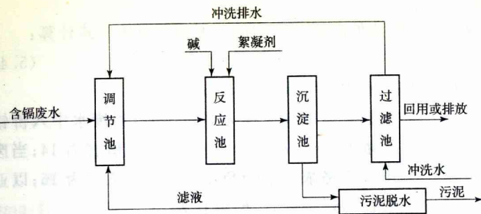
图 5.3.3 化学法处理含镉废水的基本工艺流程
