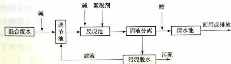
图 5.4.2 化学法处理混合废水的基本工艺流程
